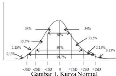
Gambar 1. Kurva Normal
