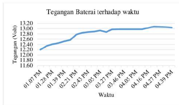
Gambar 16 Tegangan baterai terhadap waktu kontroler CMP12-10A
