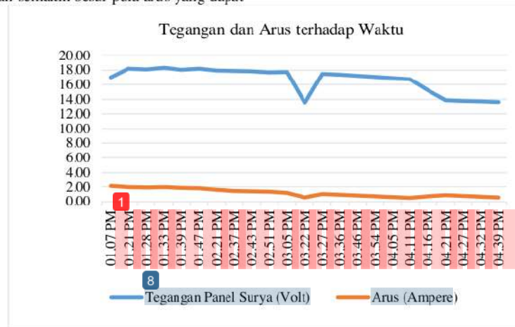
Gambar 12 Tegangan dan Arus terhadap waktu kontroler CMP12-10A
