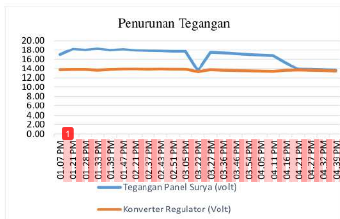
Gambar 14 Penurunan tegangan controller CMP12-10A
