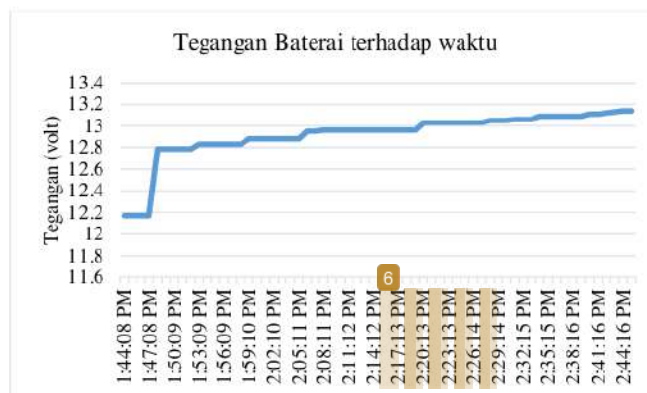
Gambar 17 Tegangan baterai terhadap waktu controller fast charging
