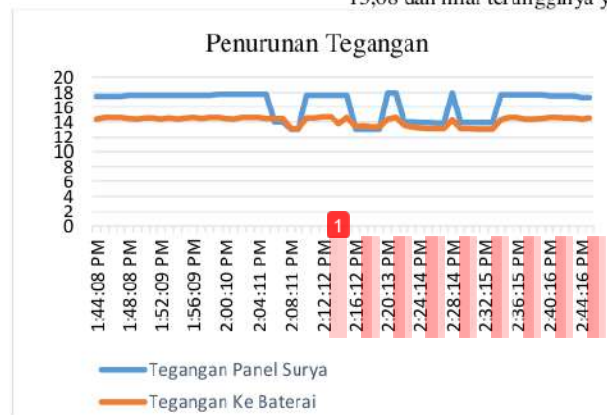
Gambar 15 Penurunan tegangan controller CMP12-10A
