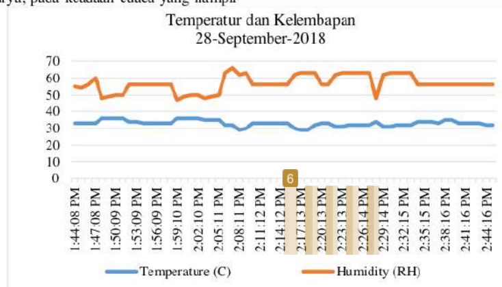
Gambar 7. Temperatur dan kelembapan data kontroler Fast Charging
