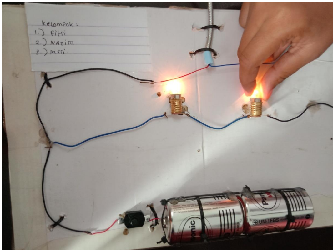
Gambar 13: Tugas siswa membuat rangkain seri parallel selama tatap muka
