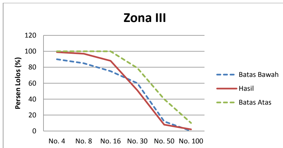
Gsmbar 4.3 Zona III Gradasi Butiran Agregat Halus
