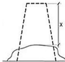
Gambar 2.5 Slump Runtuh (Sumber : Tambunan, 2015)
