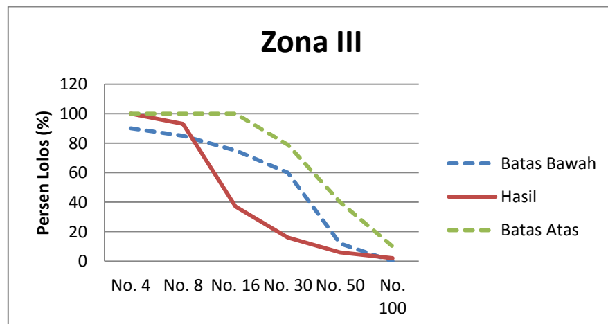
Gsmbar 4.10 Zona III Gradasi Tumbukn Cangkang Kerang
