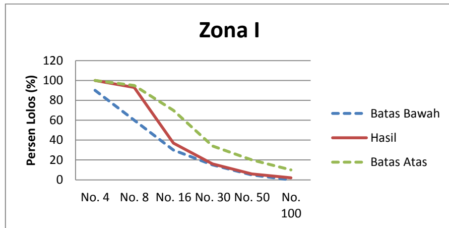
Gsmbar 4.8 Zona I Gradasi tumbukn cangkang kerang
