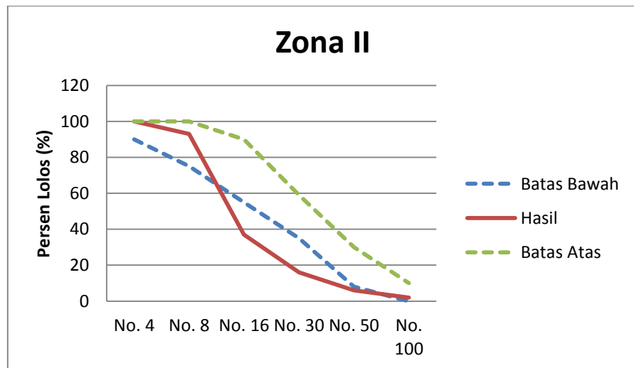
Gsmbar 4.9 Zona II Gradasi tumbukn cangkang kerang
