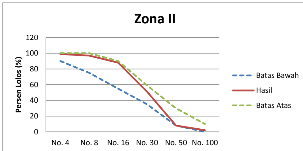
Gsmbar 4.2 Zona II Gradasi Butiran Agregat Halus
