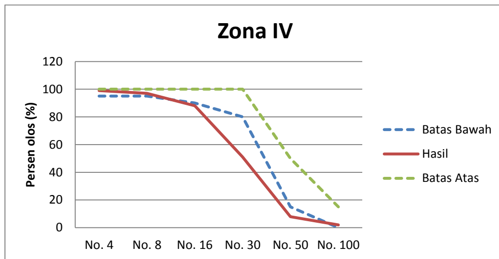
Gsmbar 4.4 Zona IV Gradasi Butiran Agregat Halus
