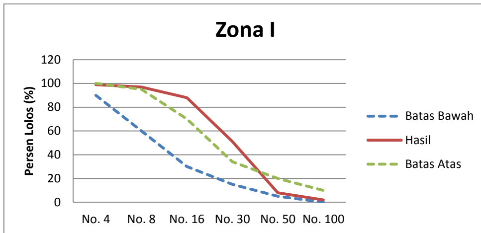
Gambar 4.1 Zona I Gradasi Butiran Agregat Halus
