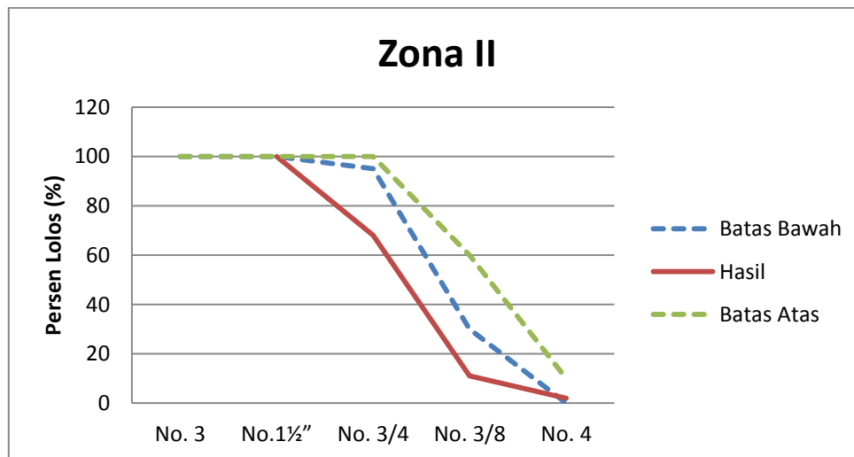
Gsmbar 4.6 Zona II Gradasi Butiran Agregat Kasar
