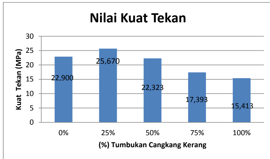
Gambar 4.13 Hasil Pengujian Kuat Tekan
