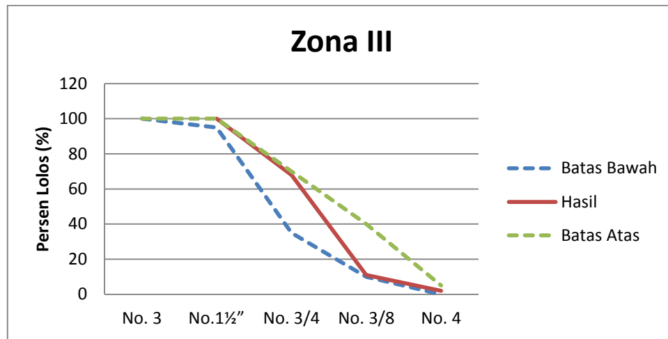
Gsmbar 4.7 Zona III Gradasi Butiran Agregat Kasar
