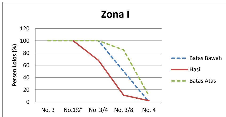
Gsmbar 4.5 Zona I Gradasi Butiran Agregat Kasar
