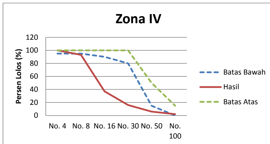
Gsmbar 4.11 Zona IV Gradasi Tumbukn Cangkang Kerang
