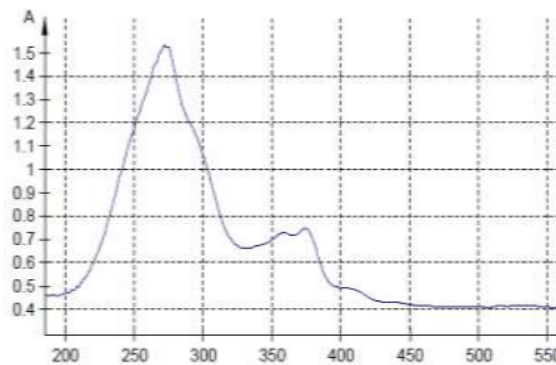
Gambar 3. Spektrum UV-Vis isolat F4
