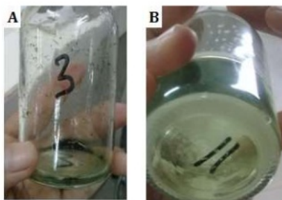
Gambar 1. Endapan yang terbentuk (a) fraksi 2 (b) fraksi 4
