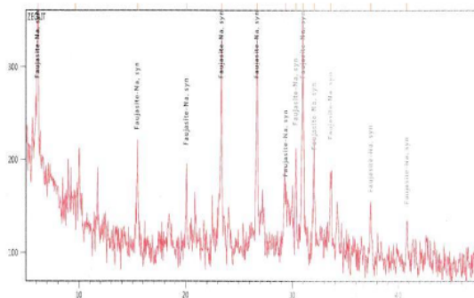
Gambar 1. Karakterisasi zeolit menggunakan XRD
