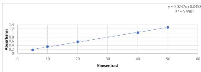
Gambar 1. Kurva kalibrasi merkuri
