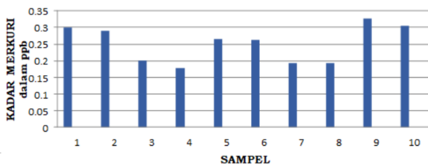
Gambar 2. Grafik kadar merkuri dalam krim pemutih.
