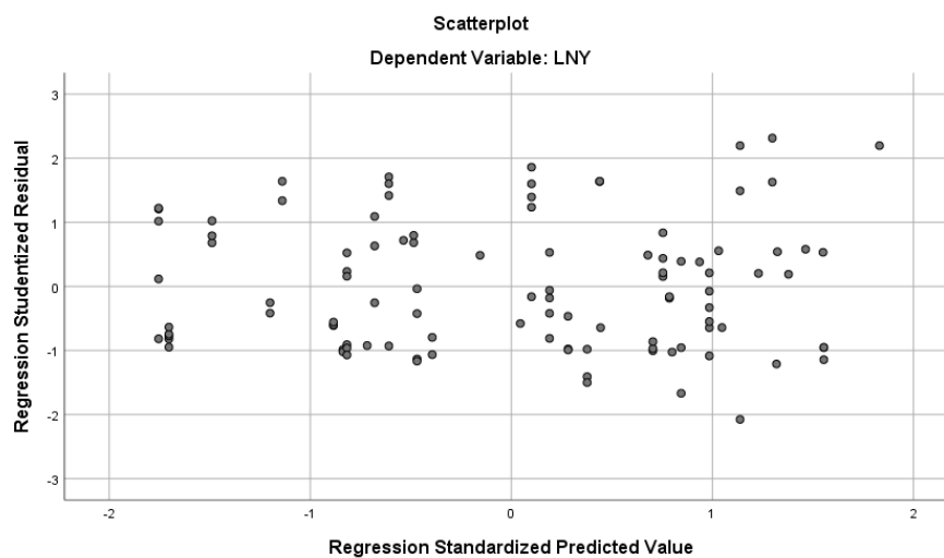
Grafik 5. 1 : Hasil Uji Heteroskedastisitas
